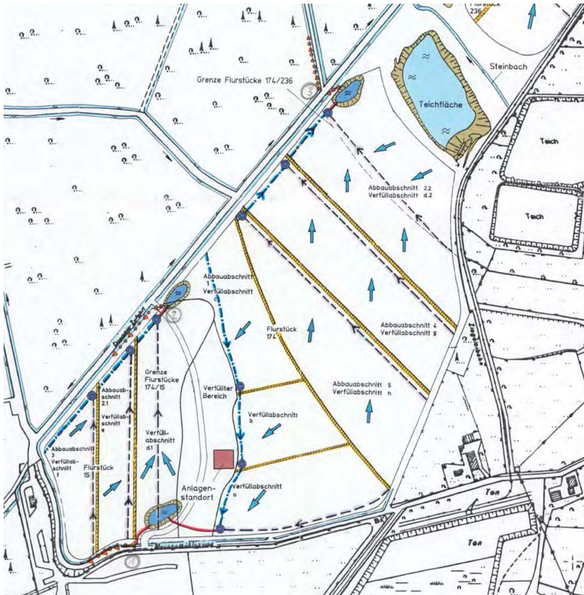
Abbildung 16: Anordnung der Abbaubabschnitte und Verfüllbereiche mit Darstellung der Trennrippen (braun) sowie Entwässerung (blau), Planung 1999, unmaßstäbliche Darstellung; Anlage 4.5 in [27].
