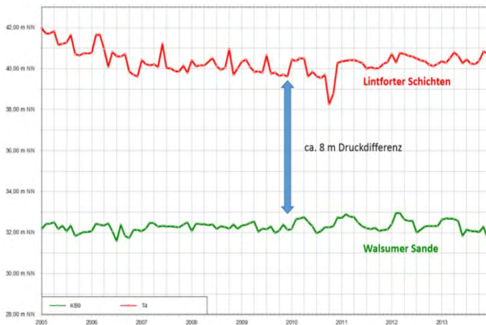
Abbildung 12: Hydraulische Druckhöhen der Messstelle T4 (Lintforter Schichten) und KB9 (Walsumer Meeressande) [7]
