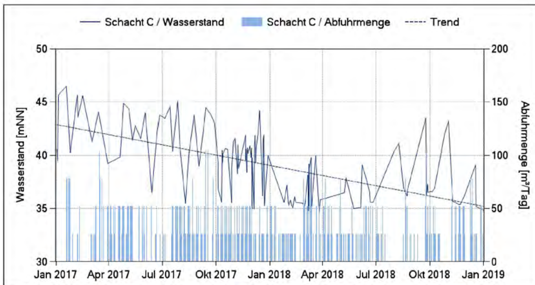
Abbildung 40: Ganglinie der Sickerwasserstände und Abfuhrmengen im Schacht C [177]
