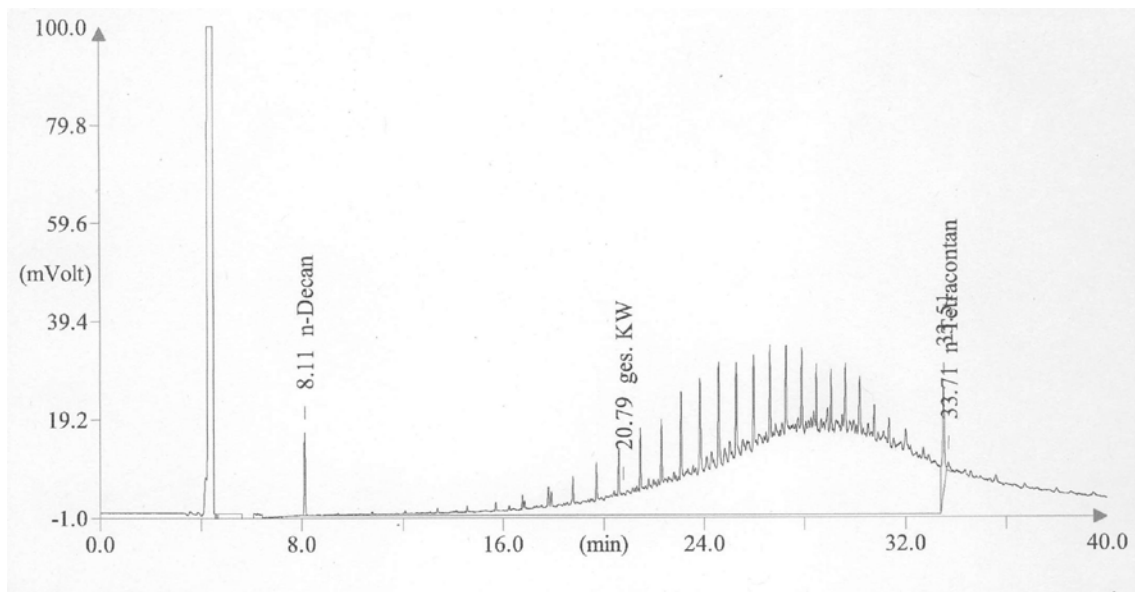
Abbildung 21: Chromatogramm der Ölpellet-Probe 1, Sieb C nach Pelletierung (Proben-Nr. 14-29193-01) [77]
