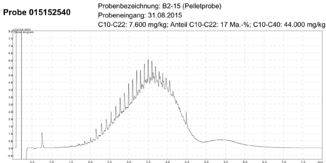
Abbildung 24: Chromatogramm einer Probe mit Ölpellet-Verdacht aus der Bohrung B2. Verändert nach [93]
