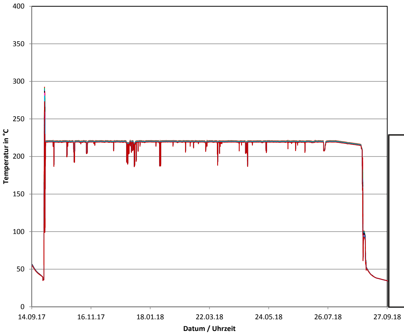
Betriebszyklus 2017/2018 Temperaturen am Speisewasserstutzen des Dampferzeugers JEA30BC001
