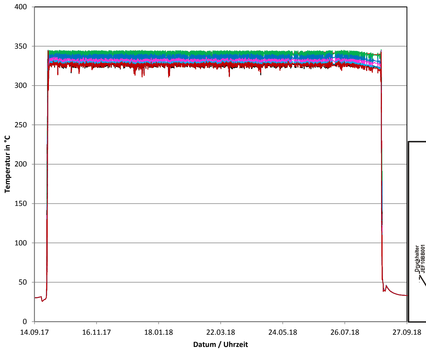
Betriebszyklus 2017/2018 Temperaturen an Volumenausgleichsleitung Mitte
