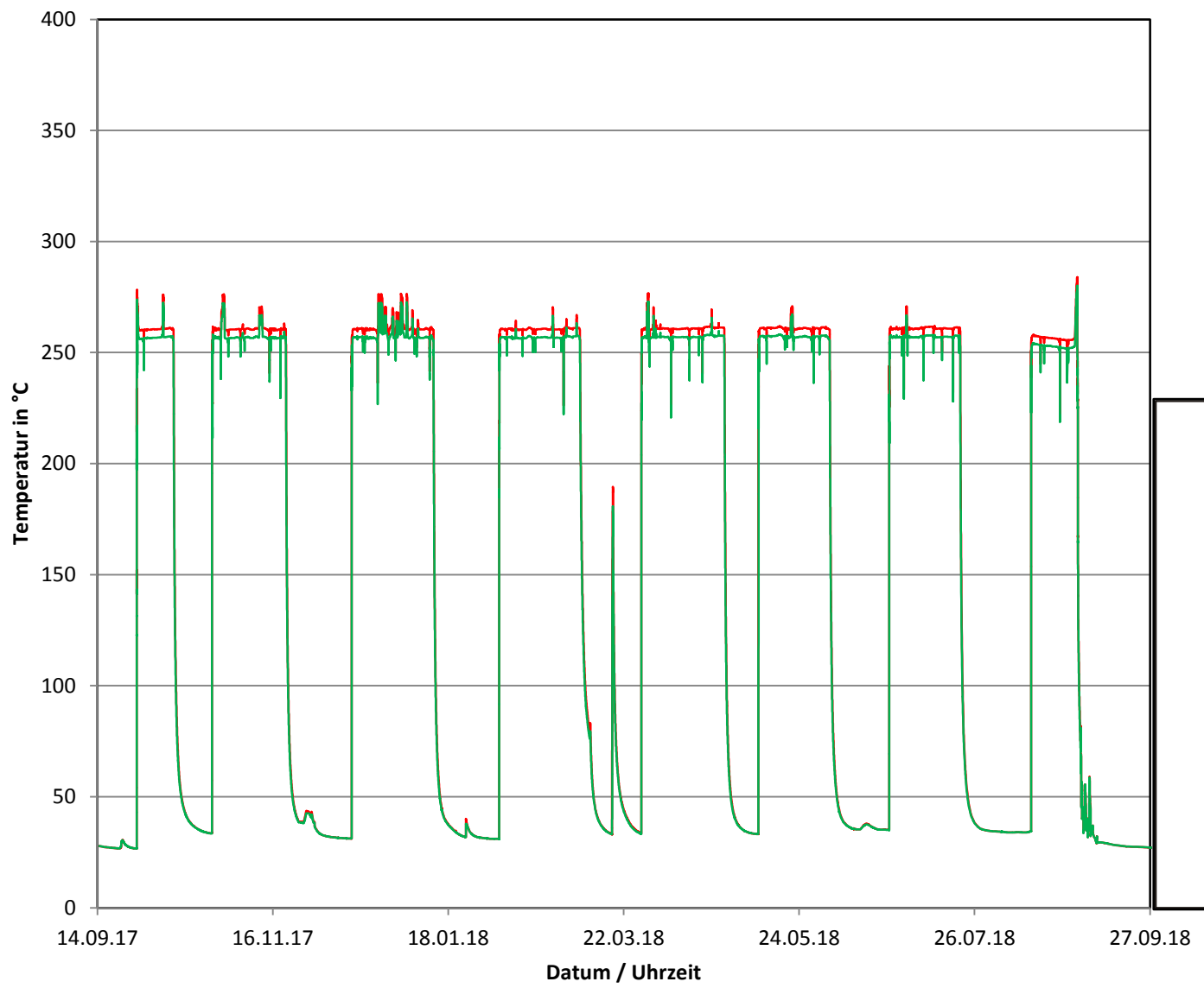
Betriebszyklus 2017/2018 Temperaturen vor Regelventil LCQ60AA001 am Abschlämmsystem LCQ60
