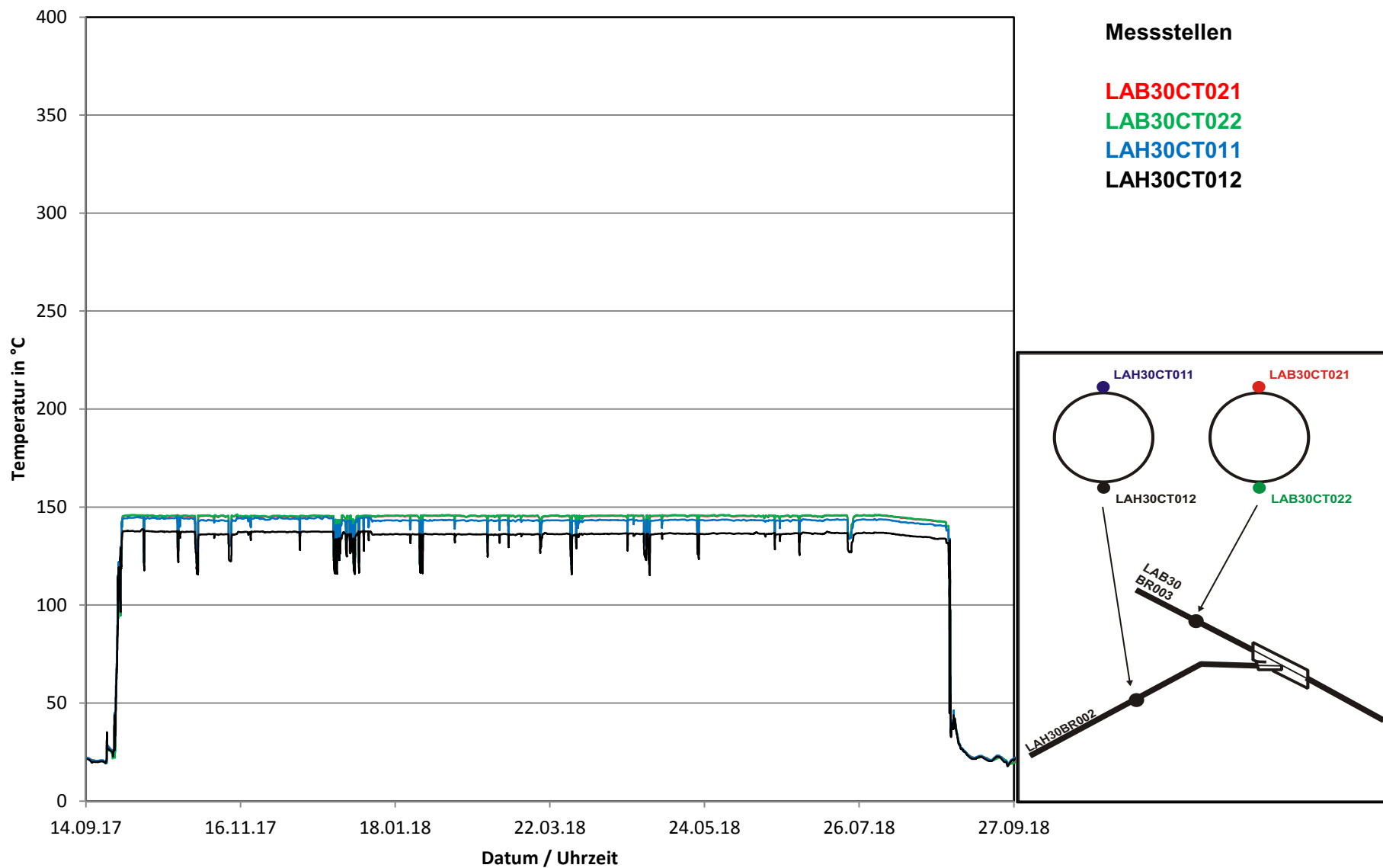
Betriebszyklus 2017/2018 Temperaturen im Bereich LAB/LAH 30
