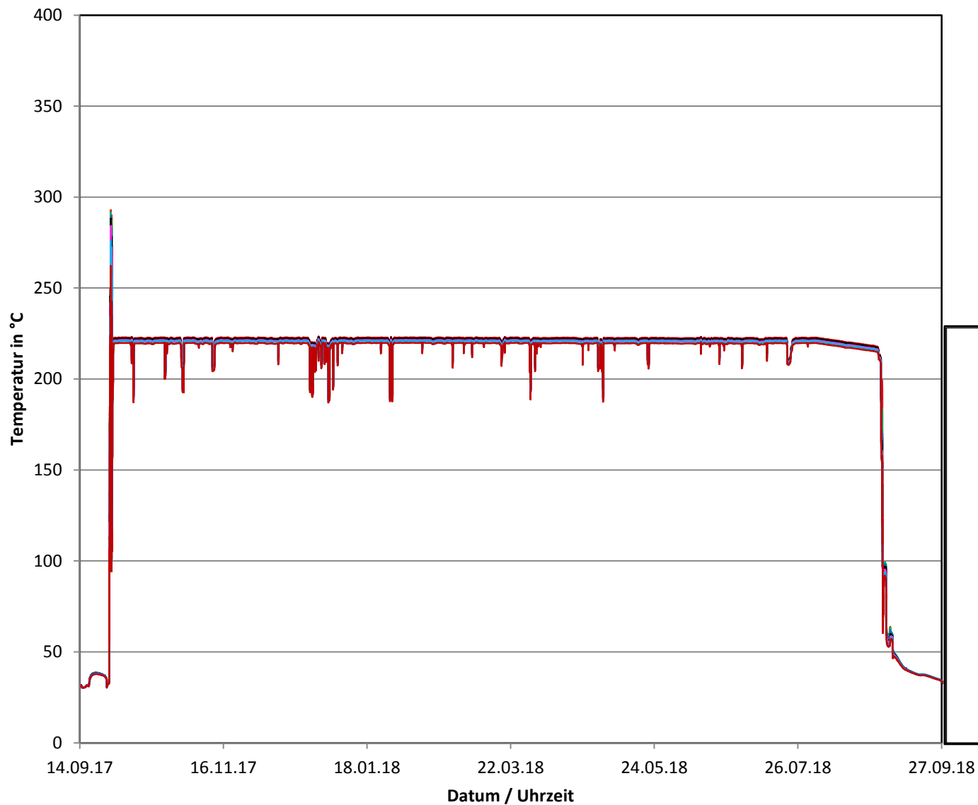
Betriebszyklus 2017/2018 Temperaturen am Speisewasserstutzen des Dampferzeugers JEA10BC001
