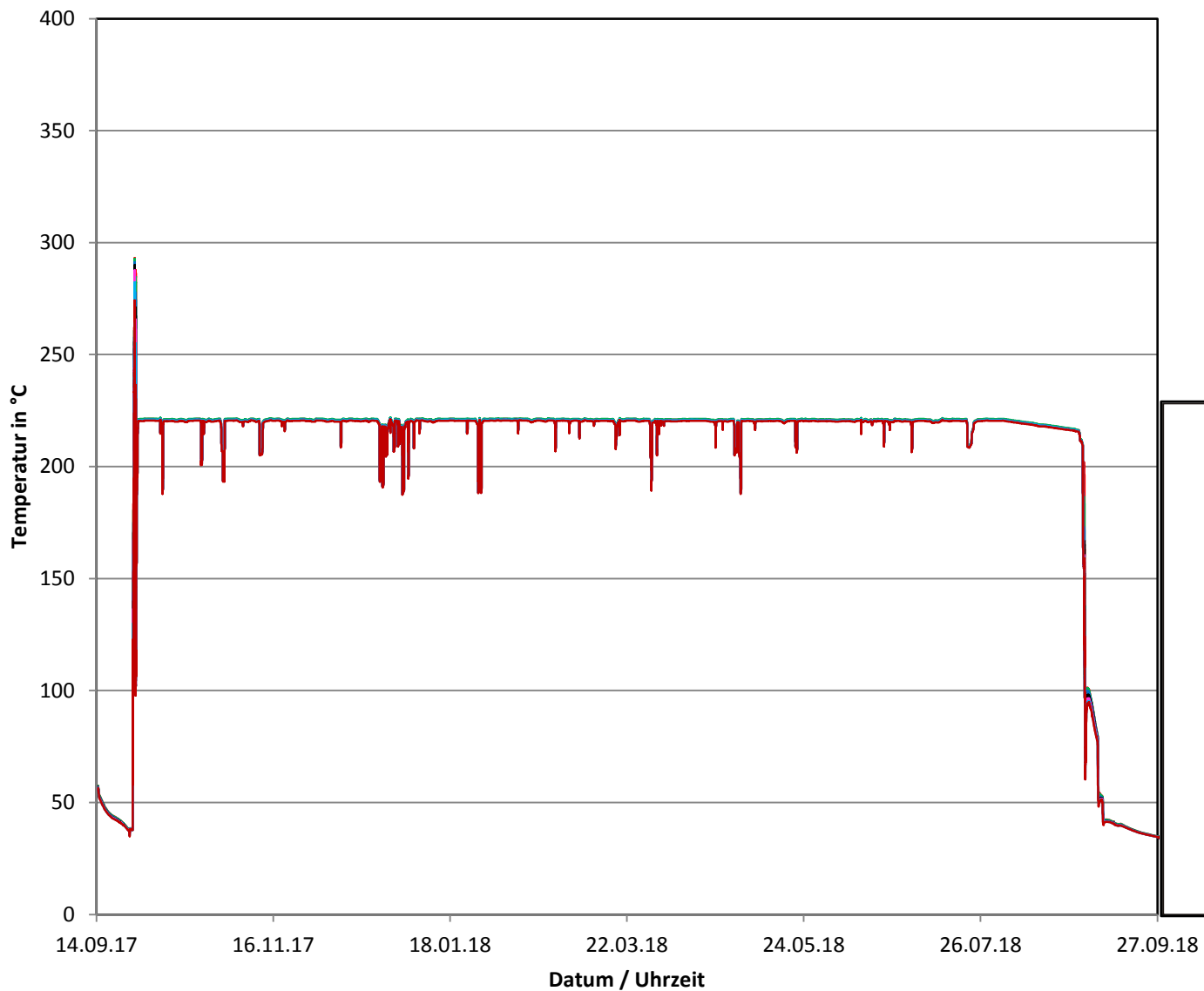
Betriebszyklus 2017/2018 Temperaturen am Speisewasserstutzen des Dampferzeugers JEA40BC001
