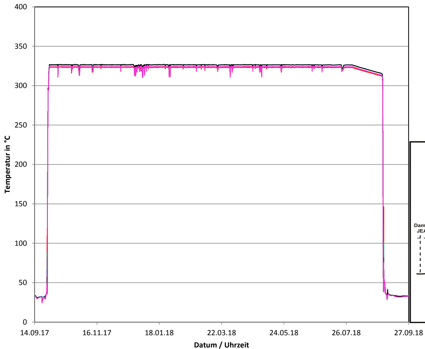
Betriebszyklus 2017/2018 Temperaturen an HKL Loop 2 nach VAL-Einbindung
