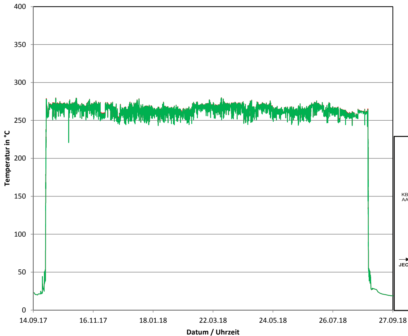
Betriebszyklus 2017/2018 Temperaturen am Einspeiseaustrittsstutzen des REKU KBA12BC001
