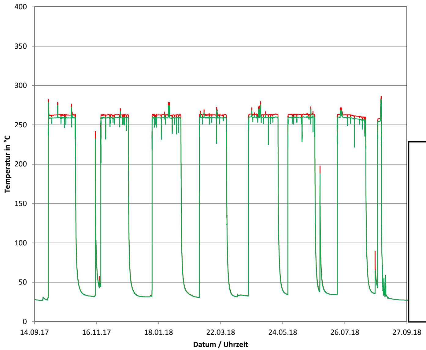
Betriebszyklus 2017/2018 Temperaturen vor Regelventil LCQ50AA001 am Abschlämmsystem LCQ50
