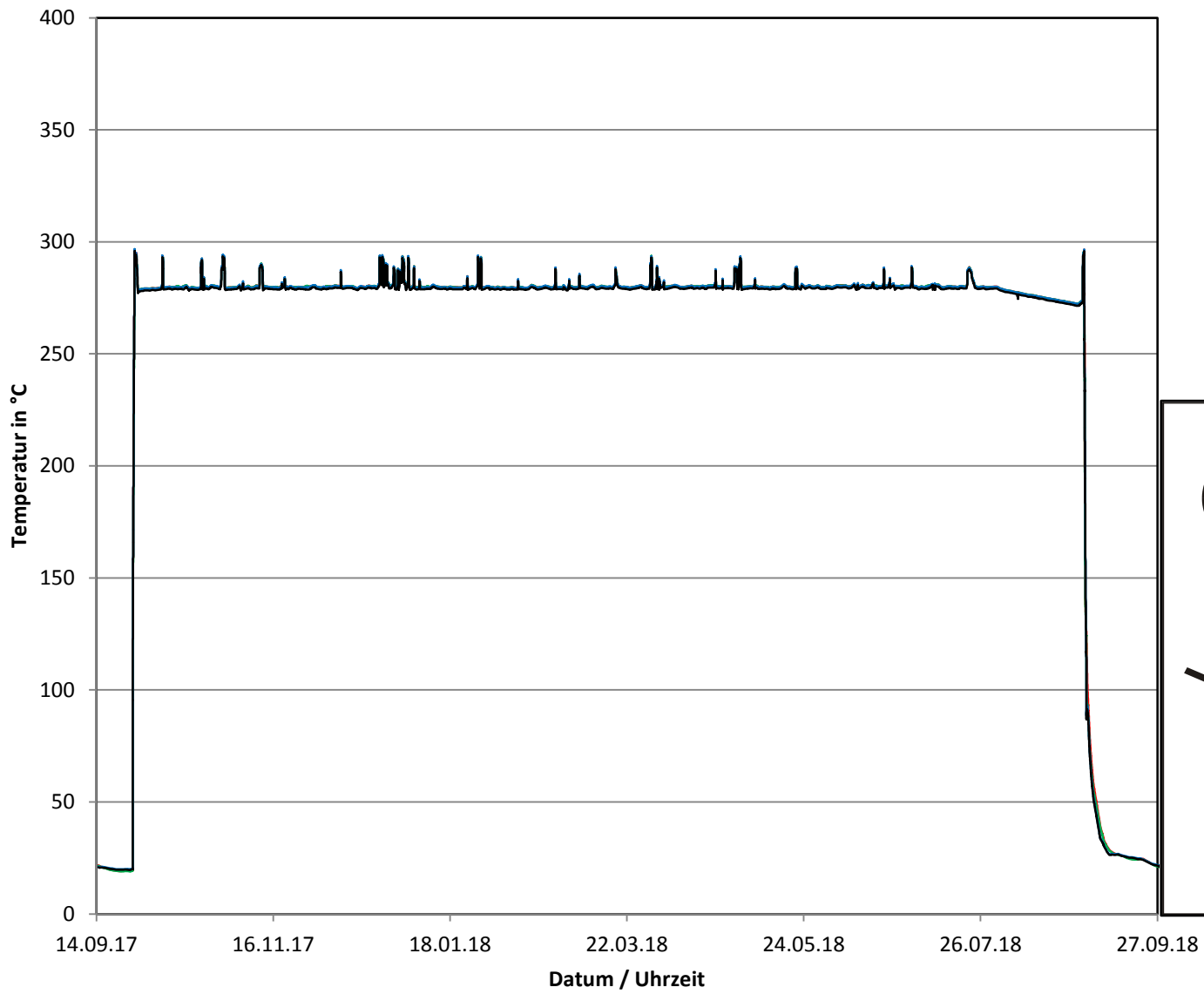
Betriebszyklus 2017/2018 Temperaturen Einbindung LBA43 in LBA40
