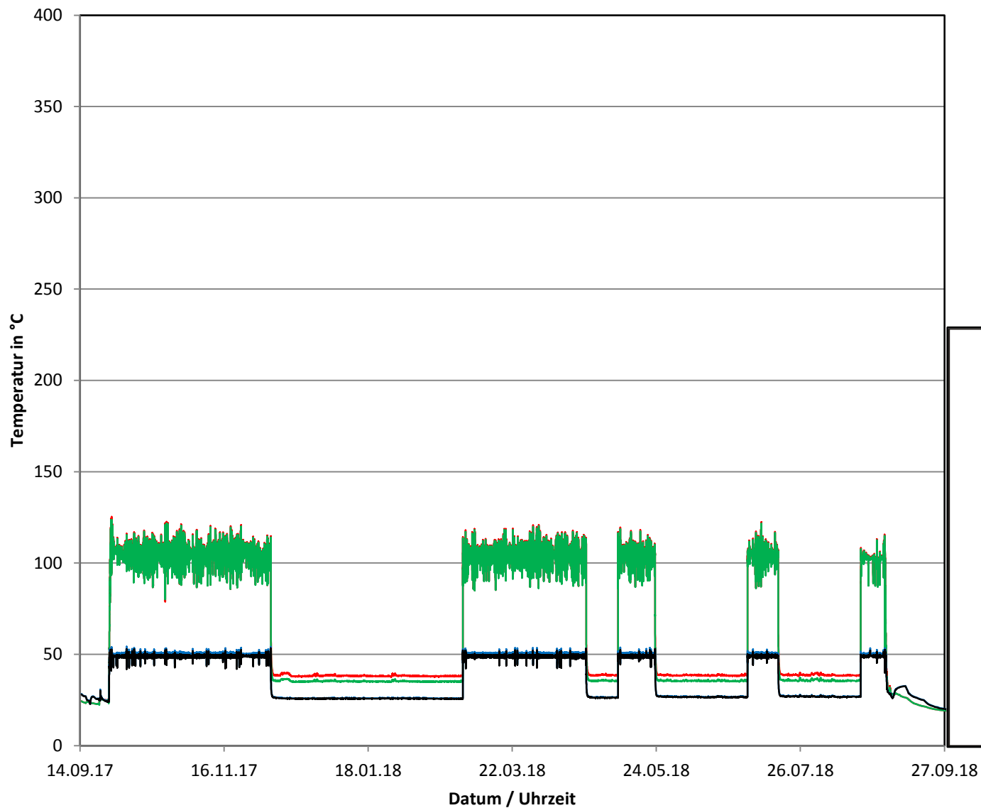
Betriebszyklus 2017/2018 Temperaturen am Ein- und Austrittsstutzen des HD-Kühlers KBA12BC002
