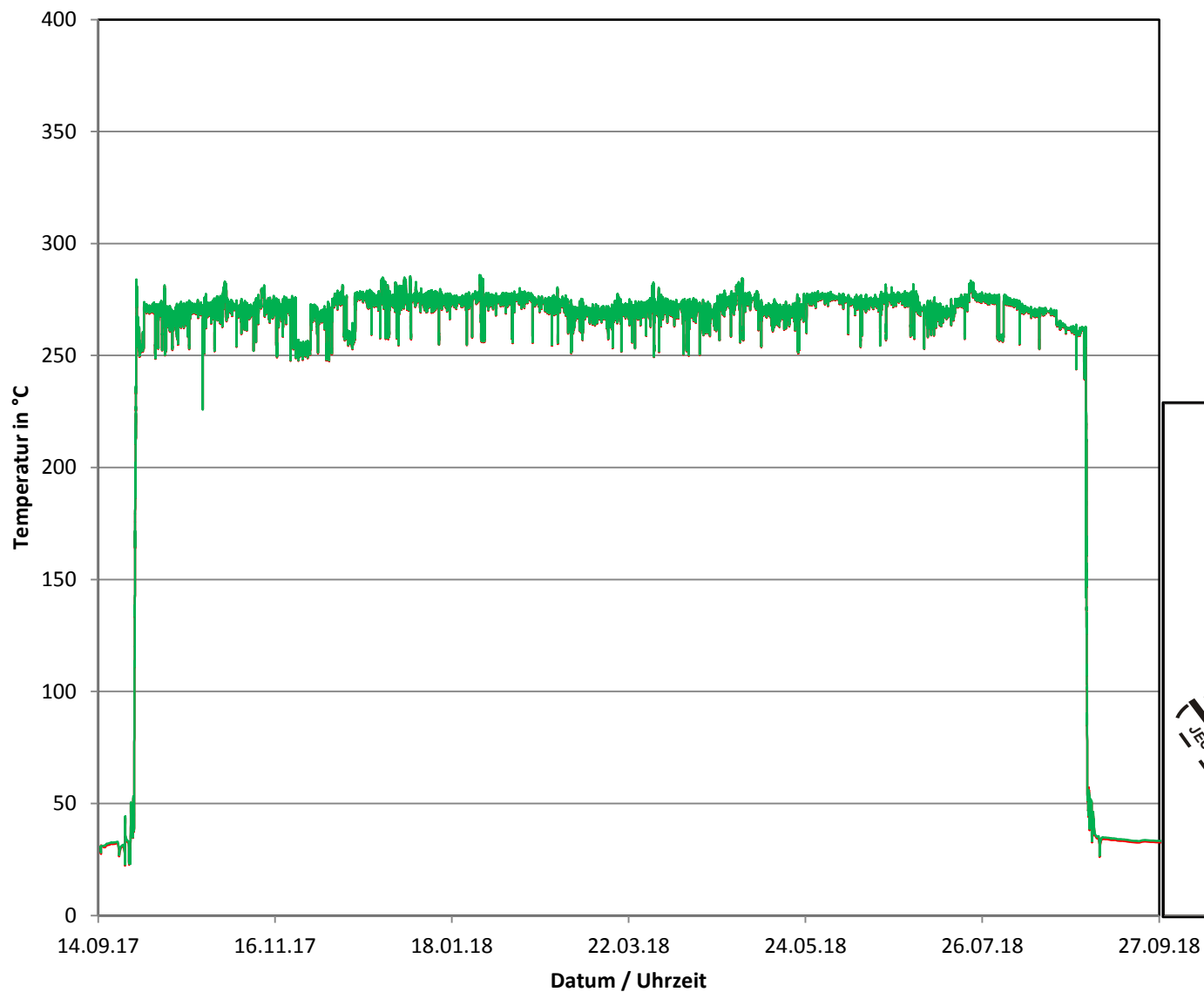
Betriebszyklus 2017/2018 Temperaturen am KBA-Einspeisestutzen an HKL Loop 2
