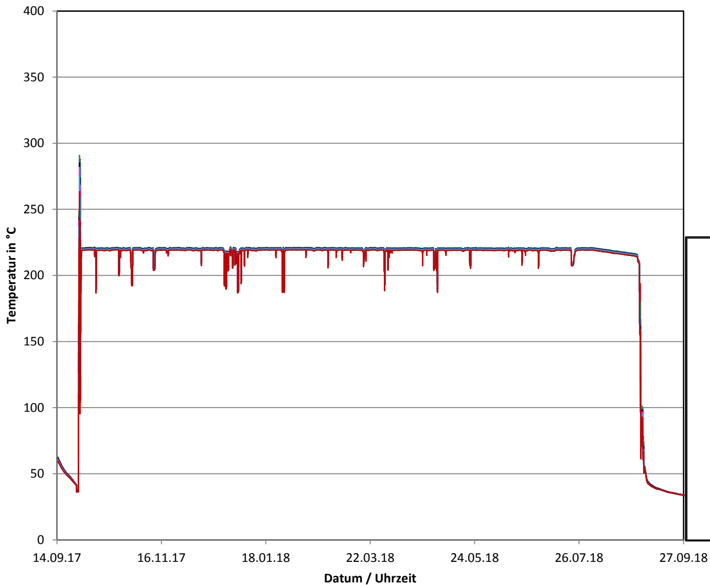
Betriebszyklus 2017/2018 Temperaturen am Speisewasserstutzen des Dampferzeugers JEA20BC001
