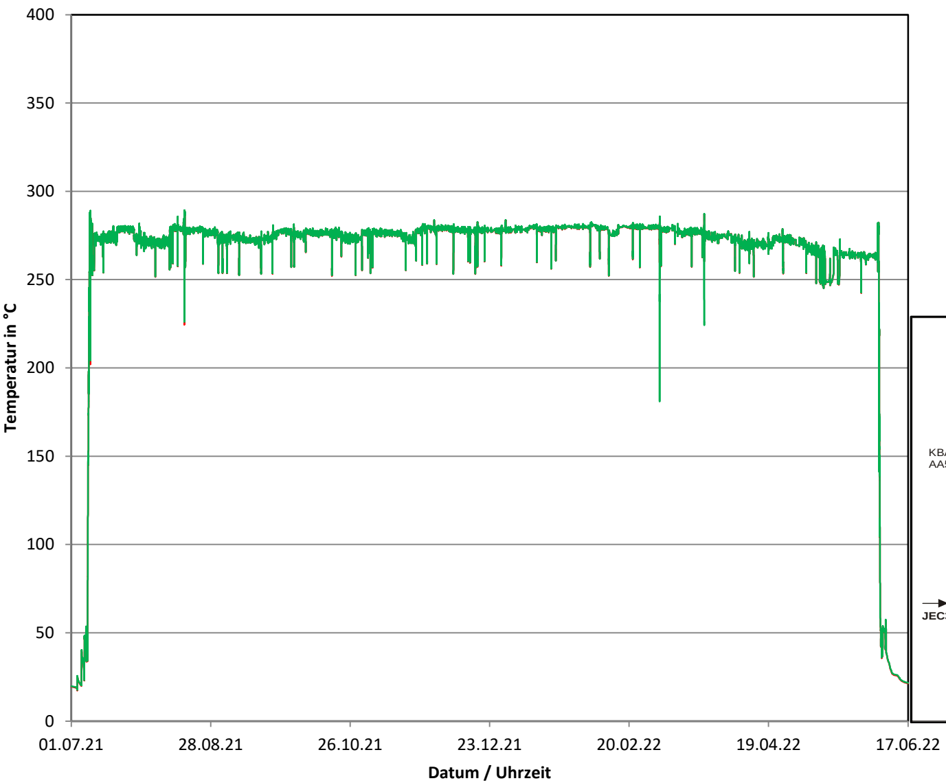
Betriebszyklus 2021/2022 Temperaturen am Einspeiseaustrittsstutzen des REKU KBA11BC001
