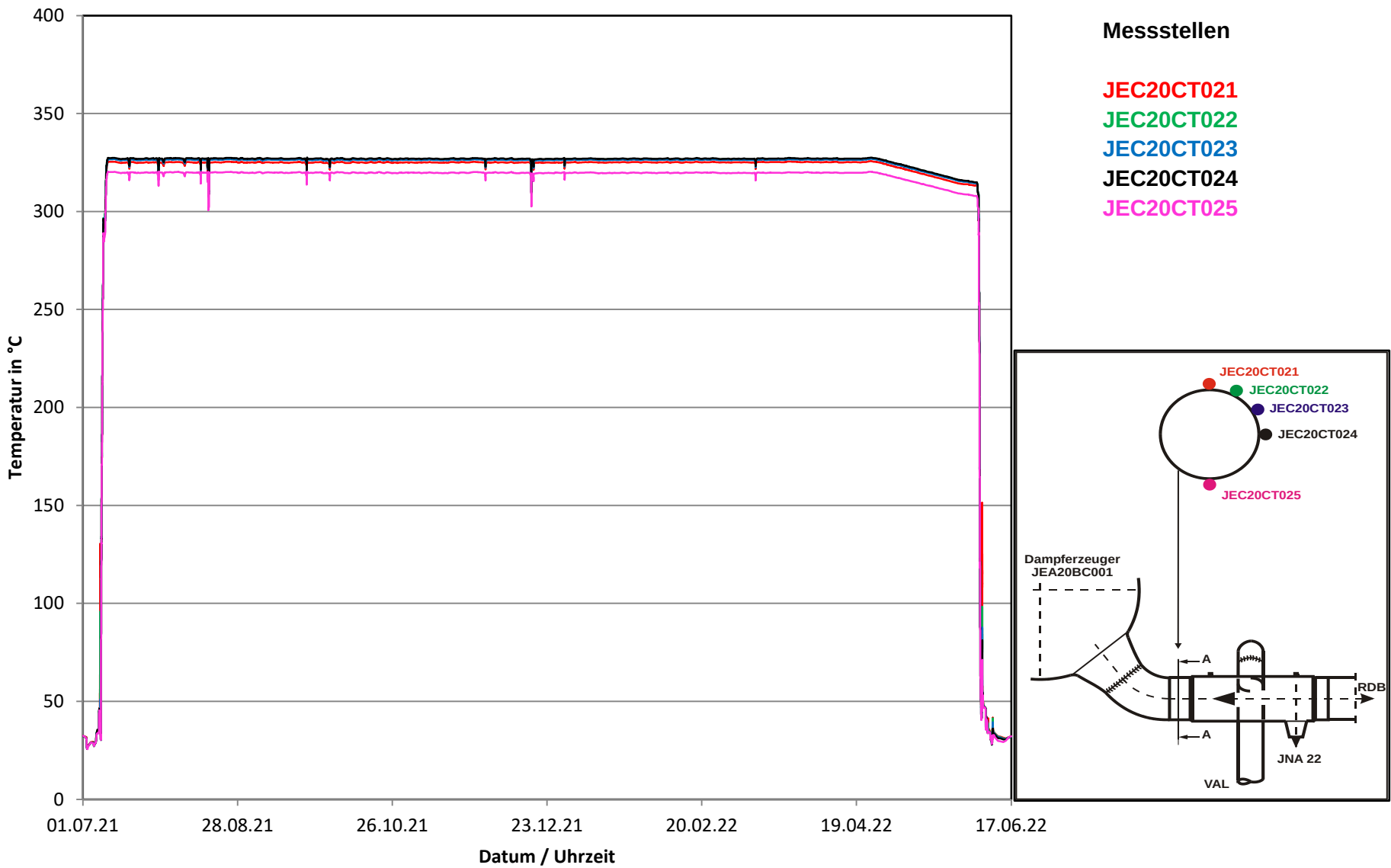
Betriebszyklus 2021/2022 Temperaturen an HKL Loop 2 nach VAL-Einbindung
