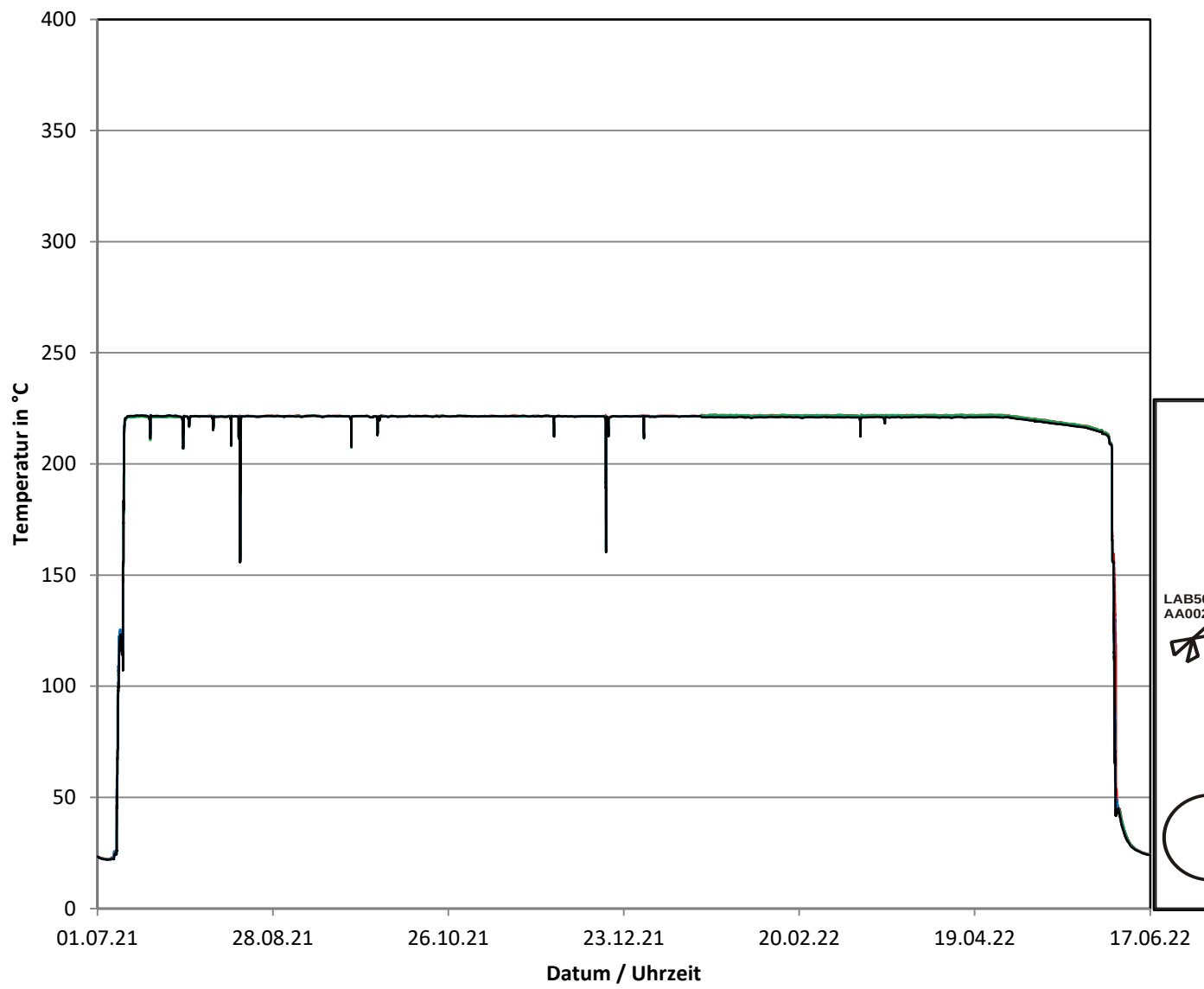
Betriebszyklus 2021/2022 Temperaturen im Bereich des Sonderformstücks LAB40/45/50
