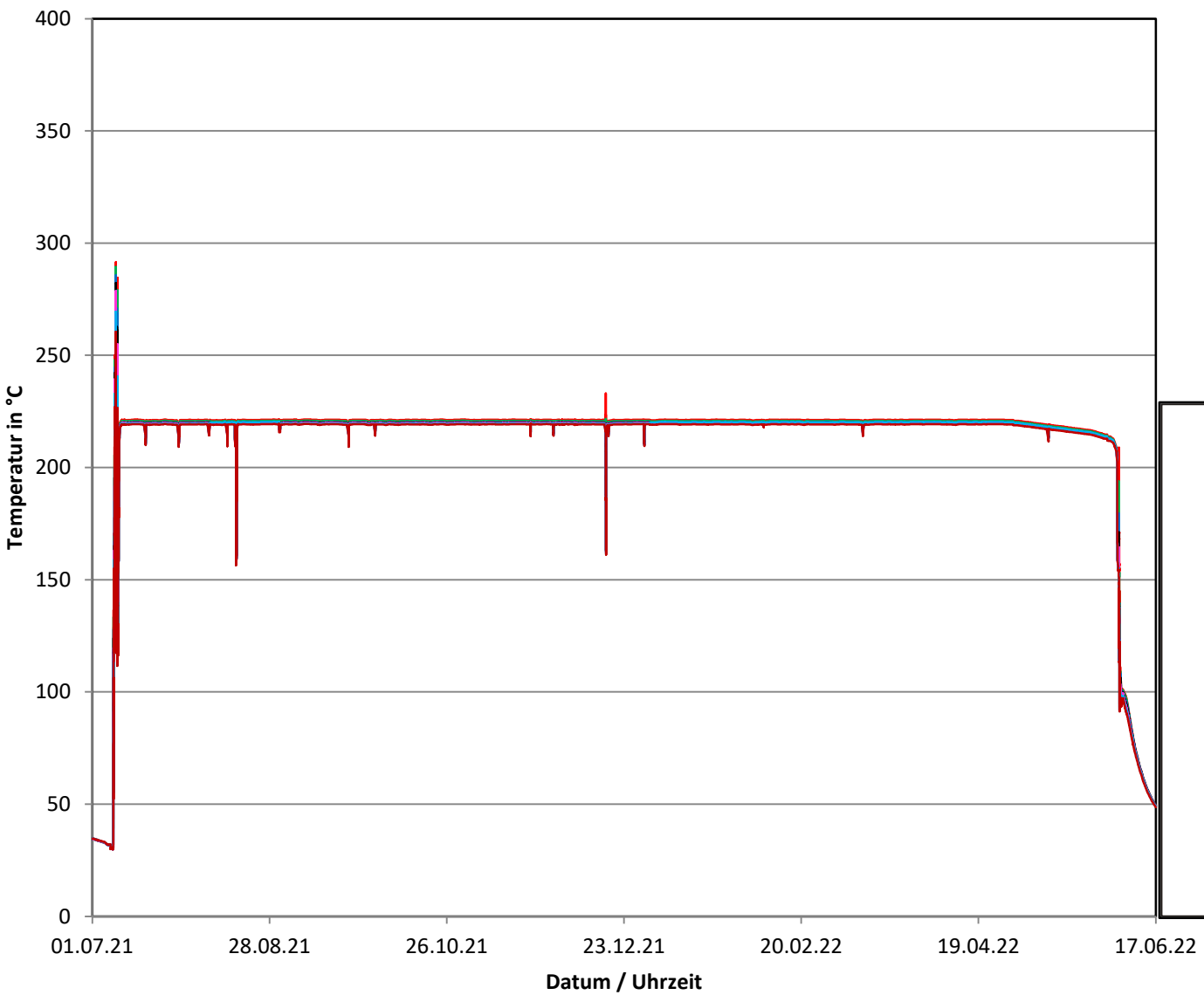
Betriebszyklus 2021/2022 Temperaturen am Speisewasserstutzen des Dampferzeugers JEA30BC001
