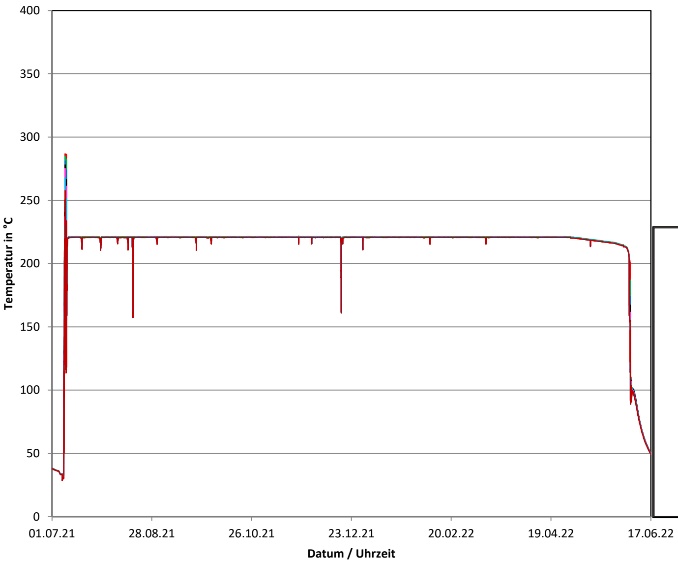
Betriebszyklus 2021/2022 Temperaturen am Speisewasserstutzen des Dampferzeugers JEA40BC001
