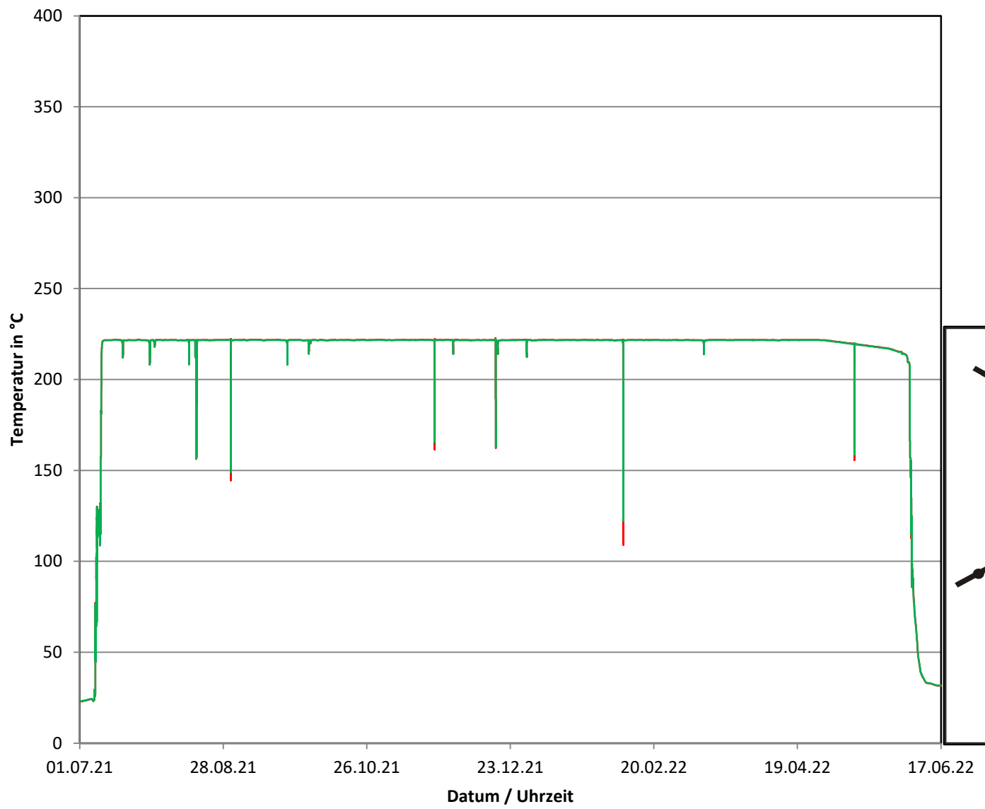
Betriebszyklus 2021/2022 Temperaturen Einbindung Schwachlastregelung Loop 2
