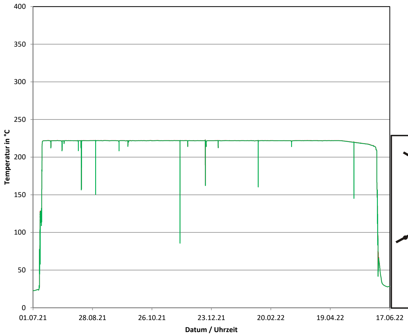
Betriebszyklus 2021/2022 Temperaturen Einbindung Schwachlastregelung Loop 1
