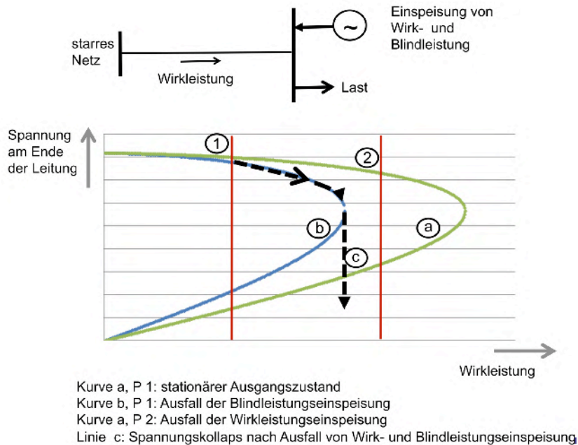
ABBILDUNG 37: VERLUST DER SPANNUNGSSTABILITÄT NACH AUSFALL VON ERZEUGUNGSEINHEITEN
