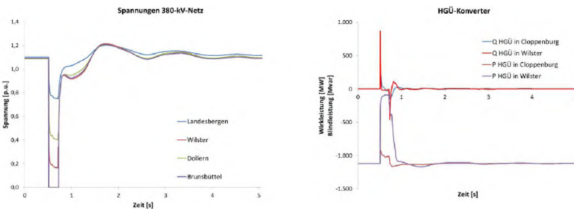
ABBILDUNG 64: 3-POLIGER KURZSCHLUSS AM UW BÜTTEL, AUSFALL EINER LEITUNG NACH WILSTER, FEHLERDAUER: 150 MS, SPANNUNGSSTÜTZUNG DURCH KONVERTER INAKTIV
