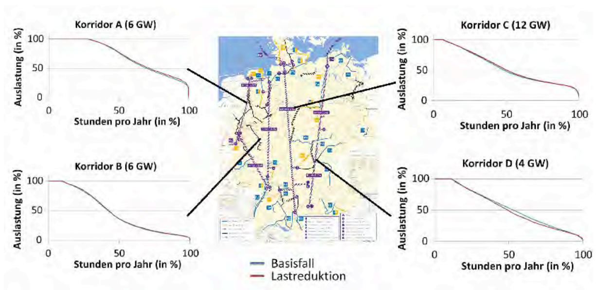
ABBILDUNG 76: GEGENÜBERSTELLUNG VON AUSLASTUNGSDAUERLINIEN DER HGÜ-KORRIDORE IM SZENARIO B 2032-BASIS UND B 2032-LASTREDUKTION
