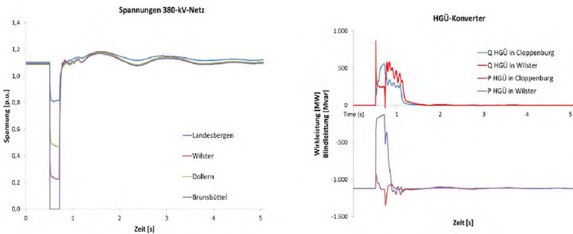
ABBILDUNG 63: 3-POLIGER KURZSCHLUSS AM UW BÜTTEL, AUSFALL EINER LEITUNG NACH WILSTER, FEHLERDAUER: 150 MS, SPANNUNGSSTÜTZUNG DURCH KONVERTER AKTIV
