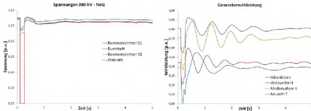
ABBILDUNG 61: 3-POLIGER KURZSCHLUSS AN HGÜ-ZULEITUNG BÜRSTADT (FEHLERDAUER: 150 MS) MIT ANSCHLIESSEN- DER ABSCHALTUNG DER HGÜ-VERBINDUNGEN CLOPPENBURG – BÜRSTADT UND WEHRENDORF – URBERACH
