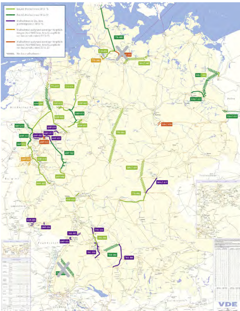
ABBILDUNG 40A: URSPRÜNGLICHE STARTNETZTOPOLOGIE MIT ENTFALLENDEN MASSNAHMEN
