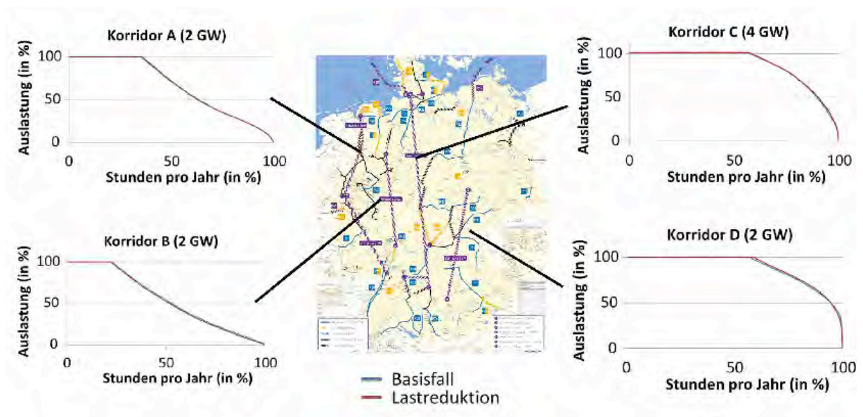
ABBILDUNG 73: GEGENÜBERSTELLUNG VON AUSLASTUNGSDAUERLINIEN DER HGÜ-KORRIDORE IM SZENARIO B 2022-BASIS UND B 2022-LASTREDUKTION
