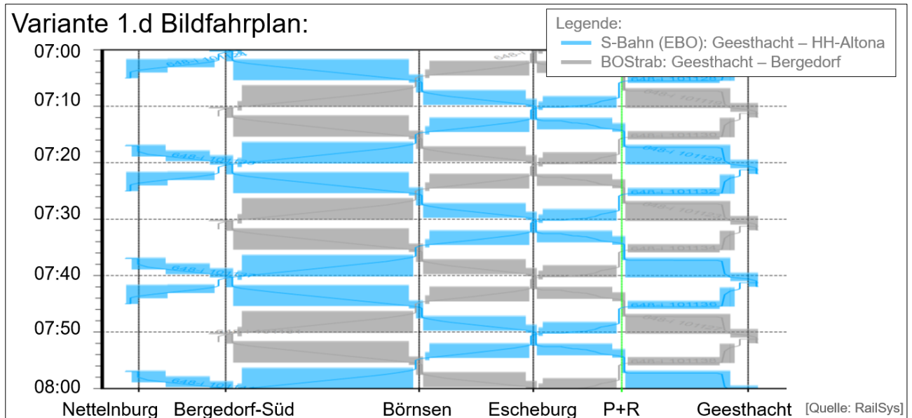
Abbildung 55: Bildfahrplan, Variante 1.d, Durchbindung S-Bahn, Auszug
