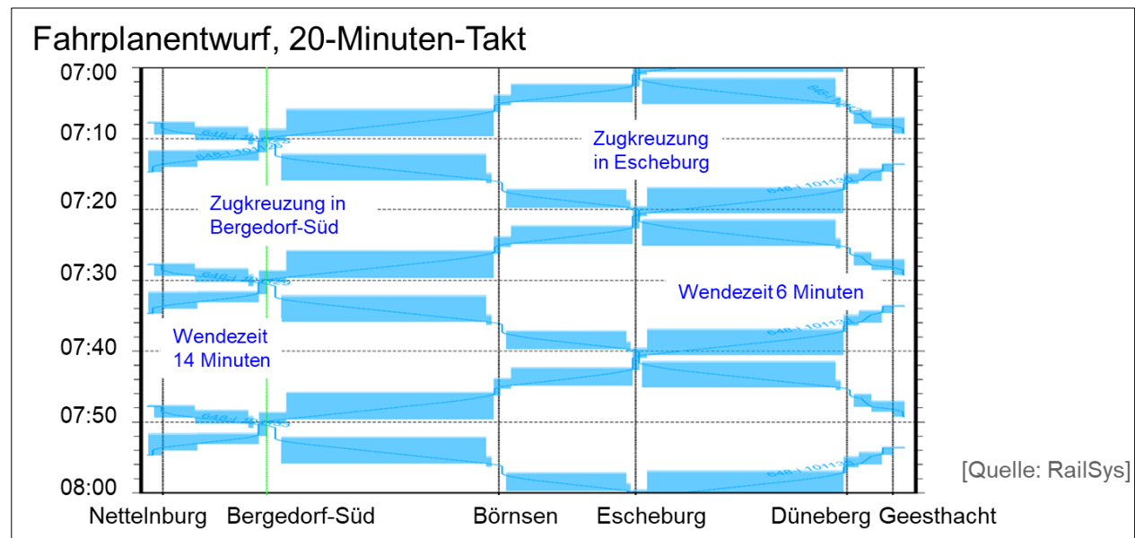
Abbildung 19: Bildfahrplan, Variante 1, EBO, Nettelnburg, Auszug Hauptverkehrszeit
