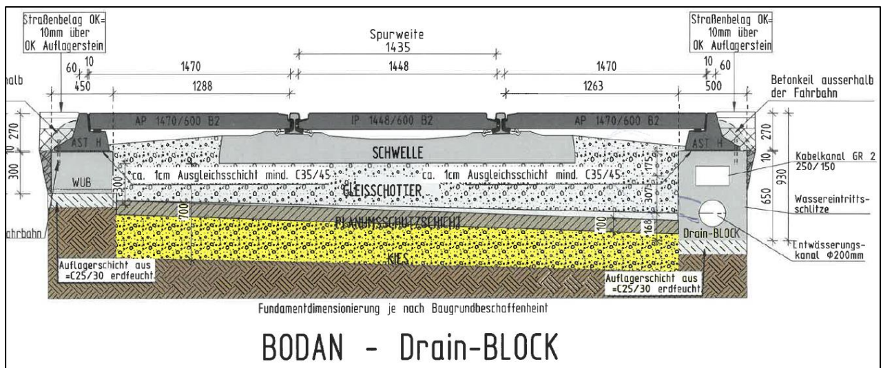
Abbildung 35: Gleiseindeckungsplatten, System Bodan [Gmundner Fertigteile GESMBH & Co.KG]
