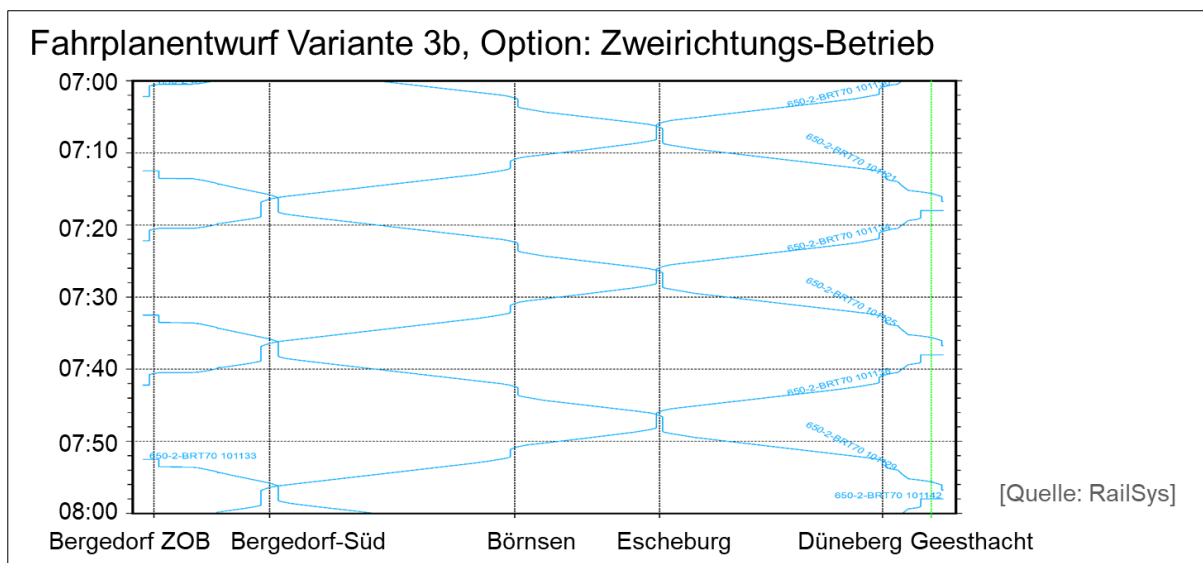
Abbildung 32: Bildfahrplan, Variante 3, BRT, Option: Zweirichtungs-Betrieb
