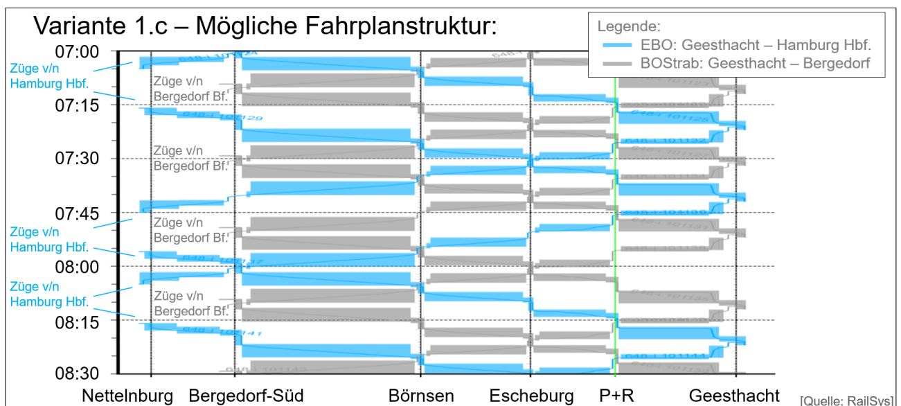
Abbildung 54: Bildfahrplan, Variante 1.c, Durchbindung Fernbahn, Auszug
