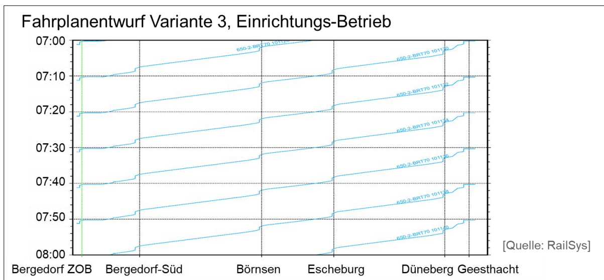
Abbildung 31: Bildfahrplan, Variante 3, BRT, Einrichtungsbetrieb
