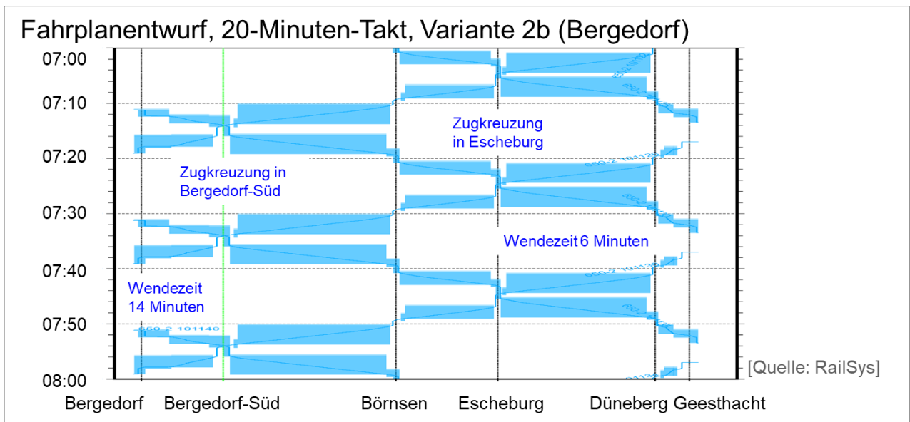
Abbildung 26: Bildfahrplan, Variante 2.b, BOStrab, Bergedorf
