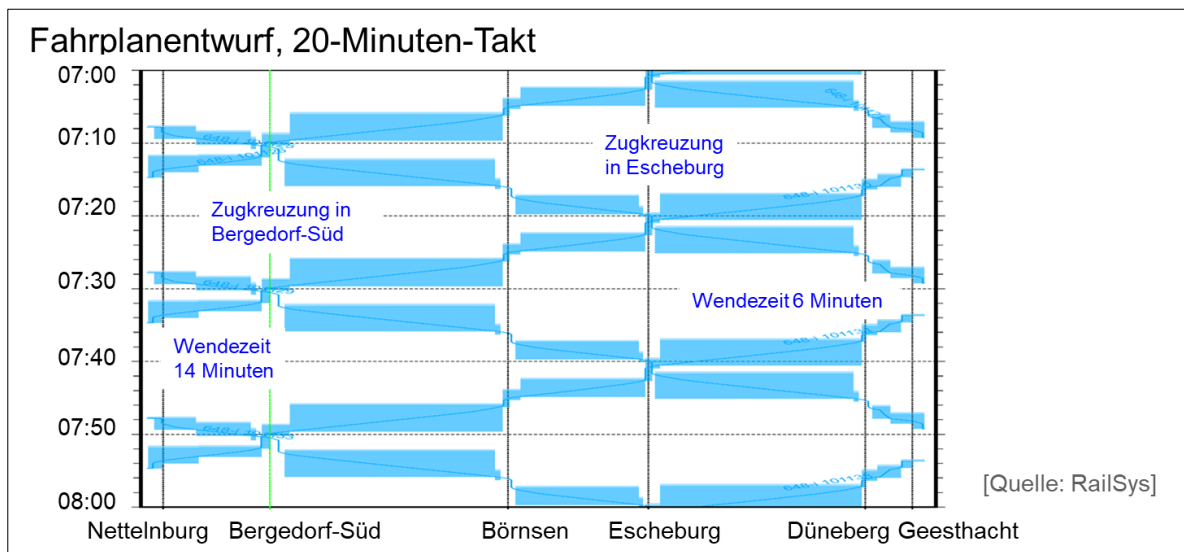
Abbildung 23: Bildfahrplan, Variante 2.a, BOStrab, Nettelburg
