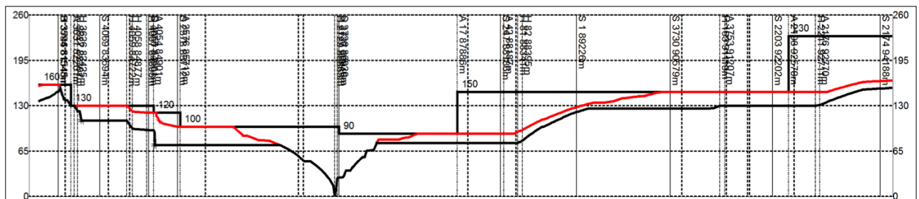
Abbildung 3: Fahrschaulinie mit Geschwindigkeitsprofil, exemplarische Strecke [Quelle: RMCon-International]
