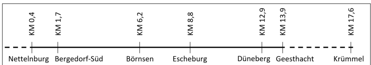
Abbildung 10: Schematische Darstellung Strecke Nettelnburg - Geesthacht [eigene Darstellung]
