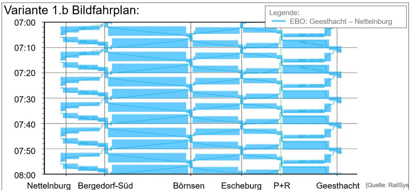
Abbildung 50: Bildfahrplan, Variante 1.b, EBO, Nettelburg, Auszug
