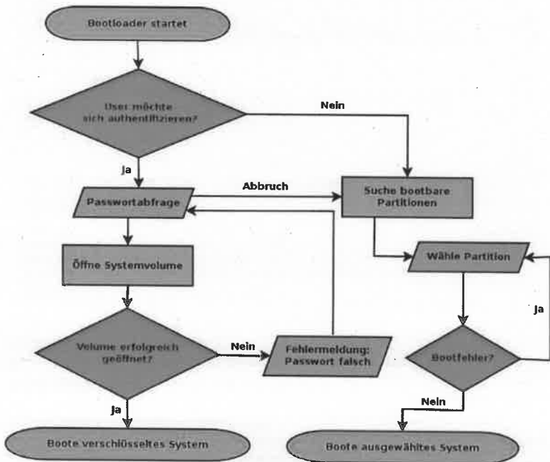
Bild 7: Flussdiagramm für Bootloader
