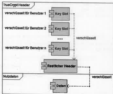
Bild 11: Key Management mittels Key Slots im Header
