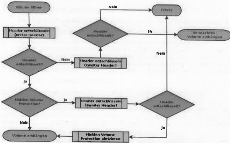
Bild 3: Flussdiagramm zum Öffnen eines Volumens
