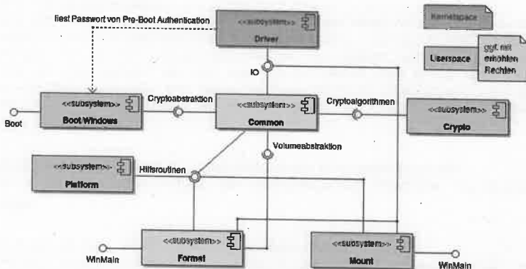
Bild 1: Übersicht der Subsystembeziehungen in Windows
