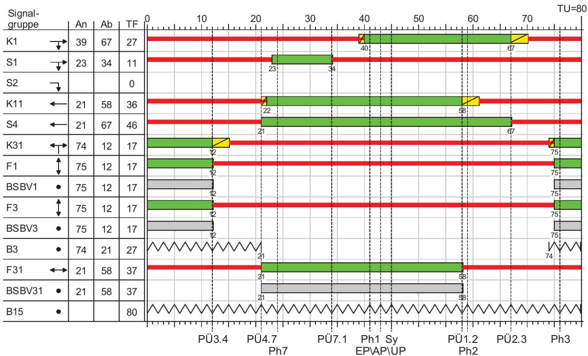
Festzeitprogramm zu P3 - mit Anforderung der Zusatzeinrichtungen für Sehbehinderte
