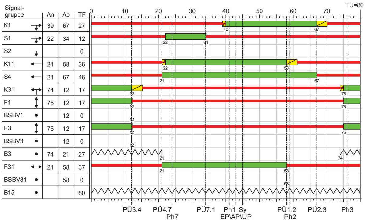
Festzeitprogramm zu P1 - ohne Anforderung der Zusatzeinrichtungen für Sehbehinderte
