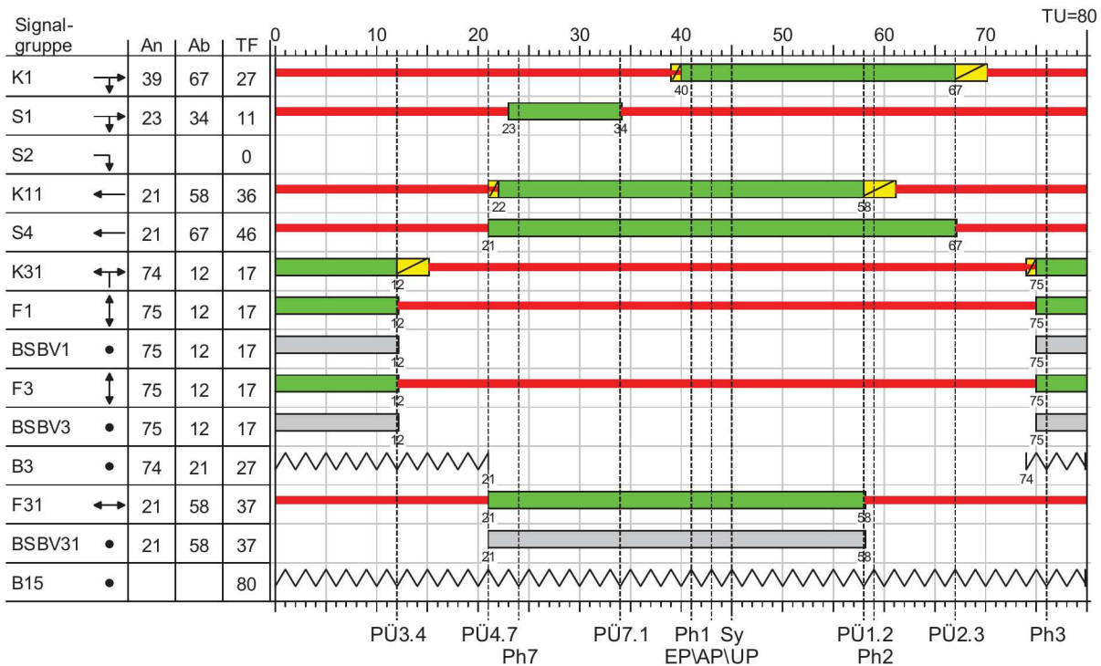
Festzeitprogramm zu P1 - mit Anforderung der Zusatzeinrichtungen für Sehbehinderte
