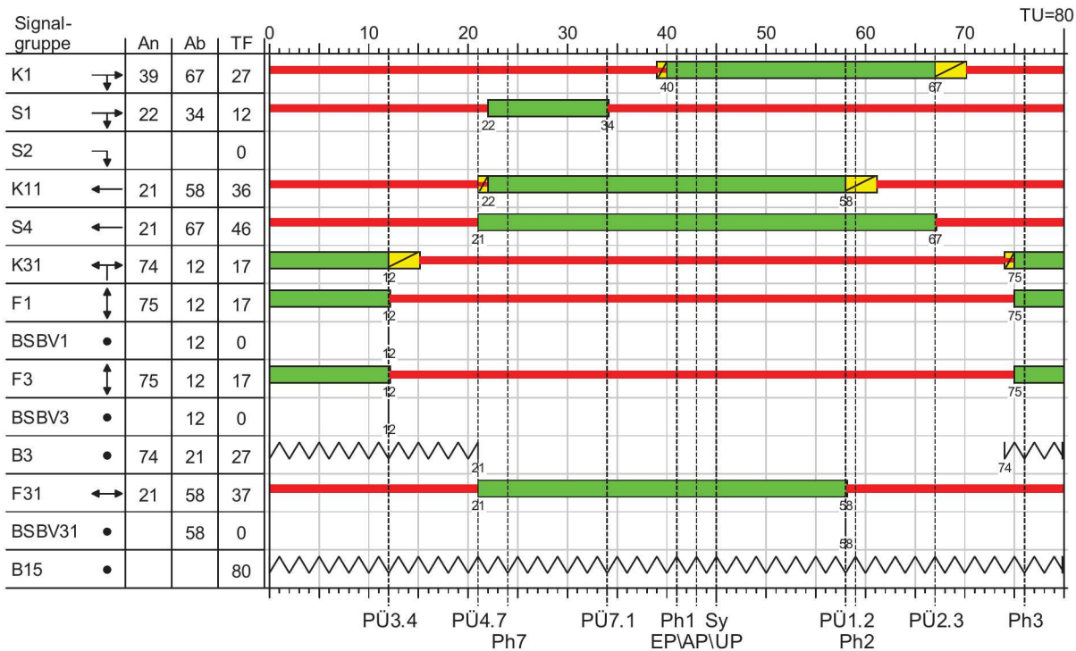
Festzeitprogramm zu P3 - ohne Anforderung der Zusatzeinrichtungen für Sehbehinderte
