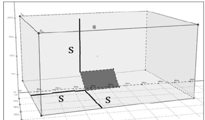
Abbildung 2.2: quaderförmiger Sicherheitsbereich
