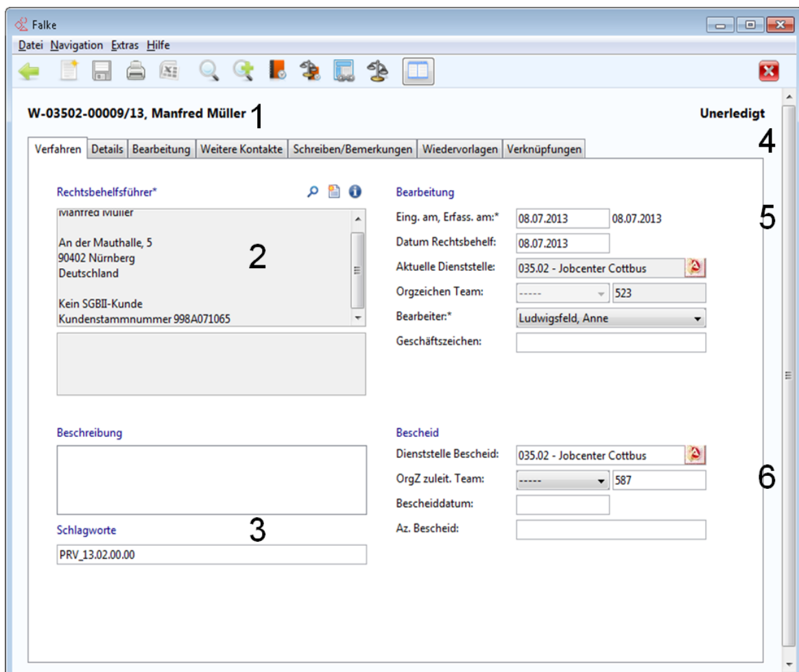
Abbildung 52 Registerkarte "Verfahren" mit den einzelnen gekennzeichneten Bereichen
