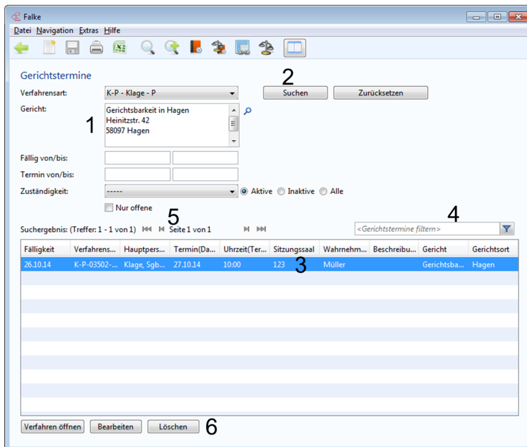
Abbildung 31 Maske „Gerichtstermine“ mit den gekennzeichneten Elementen
