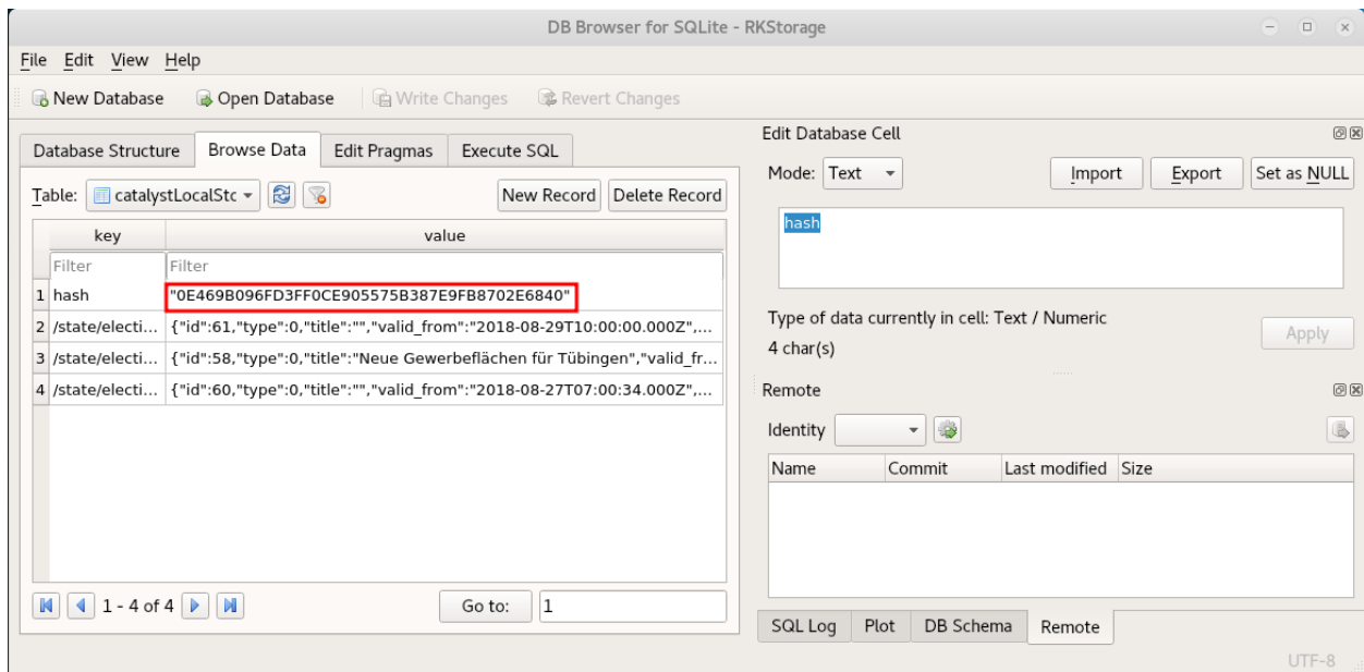
Abbildung 6.4: Der Benutzer-Hash wird in der Datenbank RKStorage im Programmverzeichnis der App gespeichert
