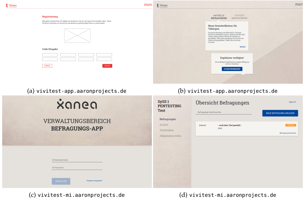
Abbildung 5.1: Webapplikationen
