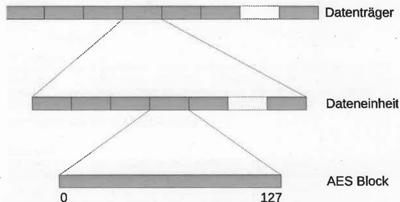
Abbildung 1.1: Aufteilung des Datenträgers im XTS Modus
