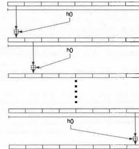
Abbildung 3.1: Mischfunktion des Zufallszahlengenerators mit der Hashfunktion h_0 unter Linux. Die Blöcke, in die der Pool aufgeteilt ist, haben die Länge des Digests der verwendeten Hashfunktion.
