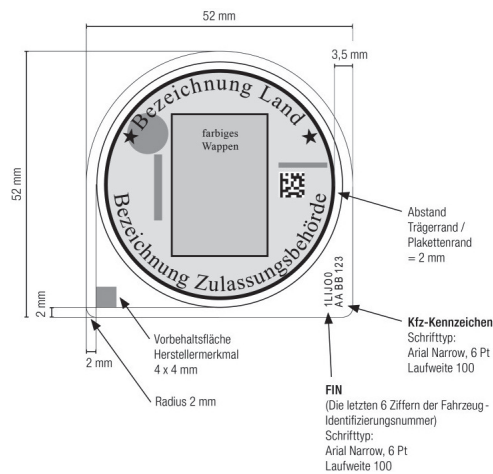
Abbildung 3: Bemaßung des Plakettenträgers
