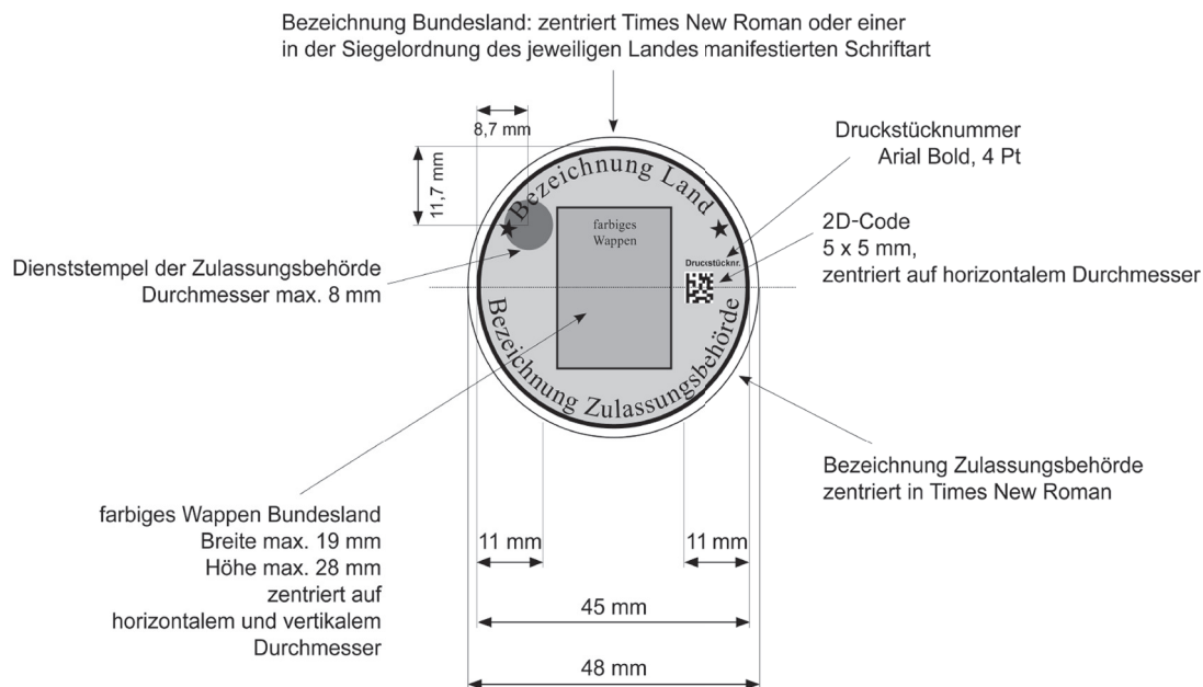
Abbildung 1: Bemaßung der Stempelplakette
