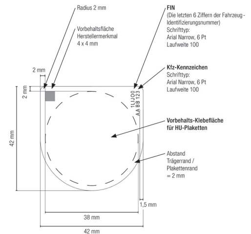
Abbildung 5: Bemaßung des HU-Plakettenträgers
