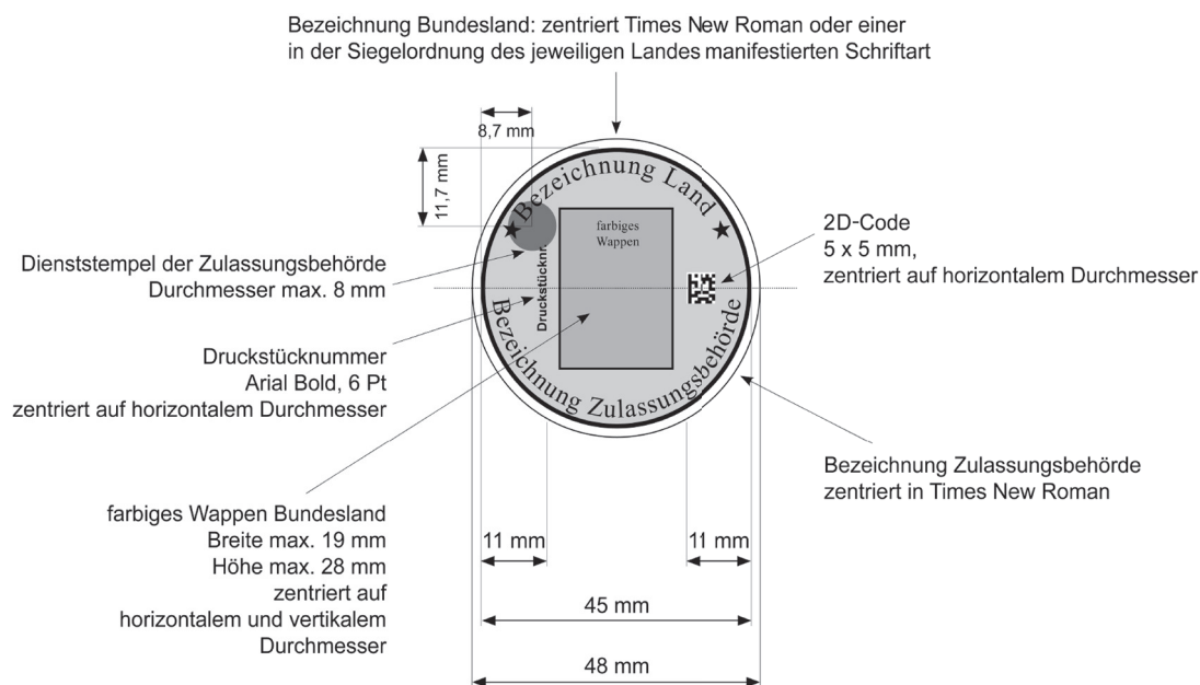
Abbildung 2: Bemaßung der Stempelplakette
