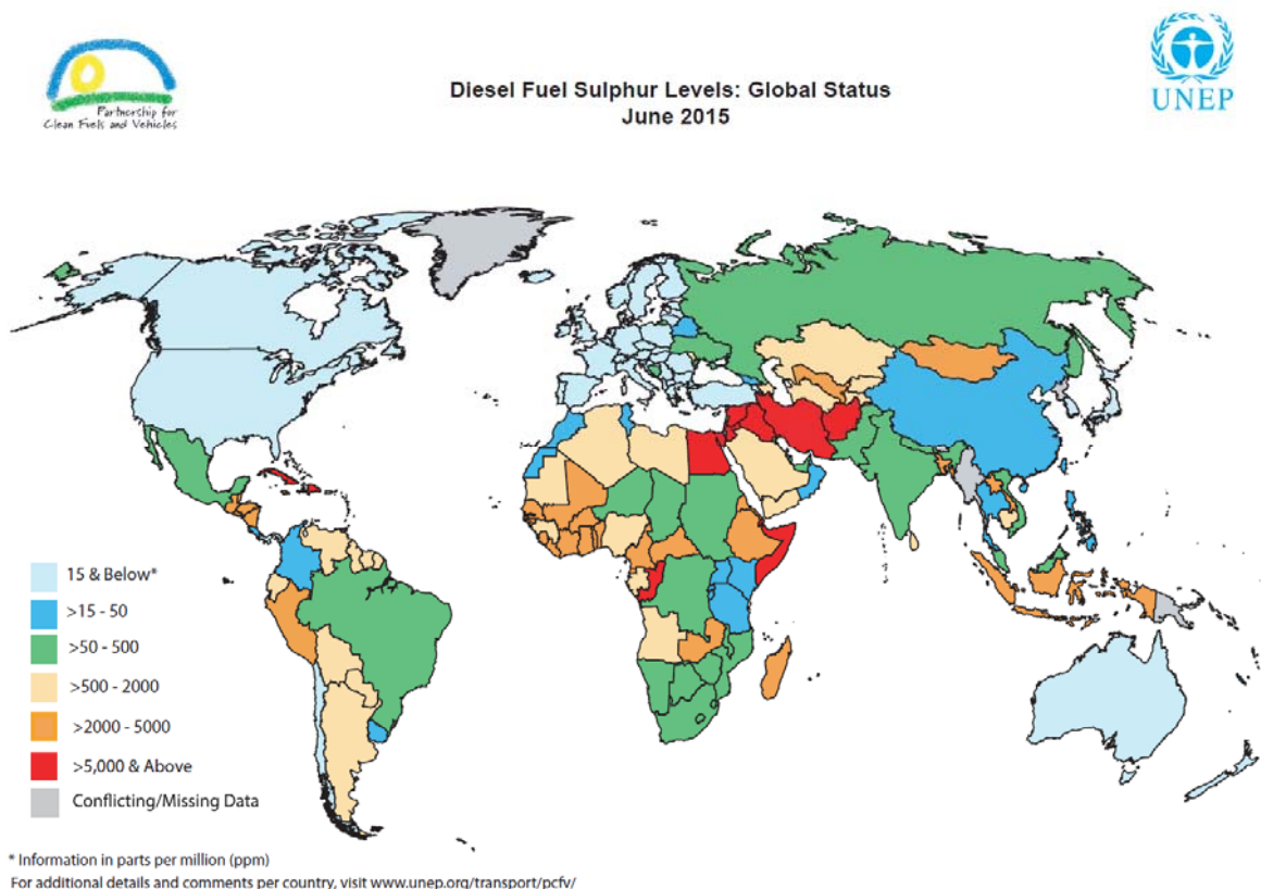
Abbildung 6: Schwefelanteil im Dieseldkraftstoff weltweit [United Nations Environment Programme, Diesel Fuel Sulphur Levels: Global Status June 2015, 2015]
